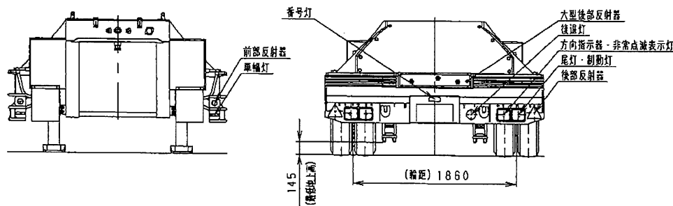
東急TL26G4E2改型 セミトレーラ外観四面図
